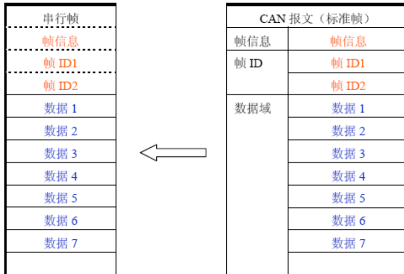
图 4.2 CAN 报文转换成串行帧 (透明方式)
